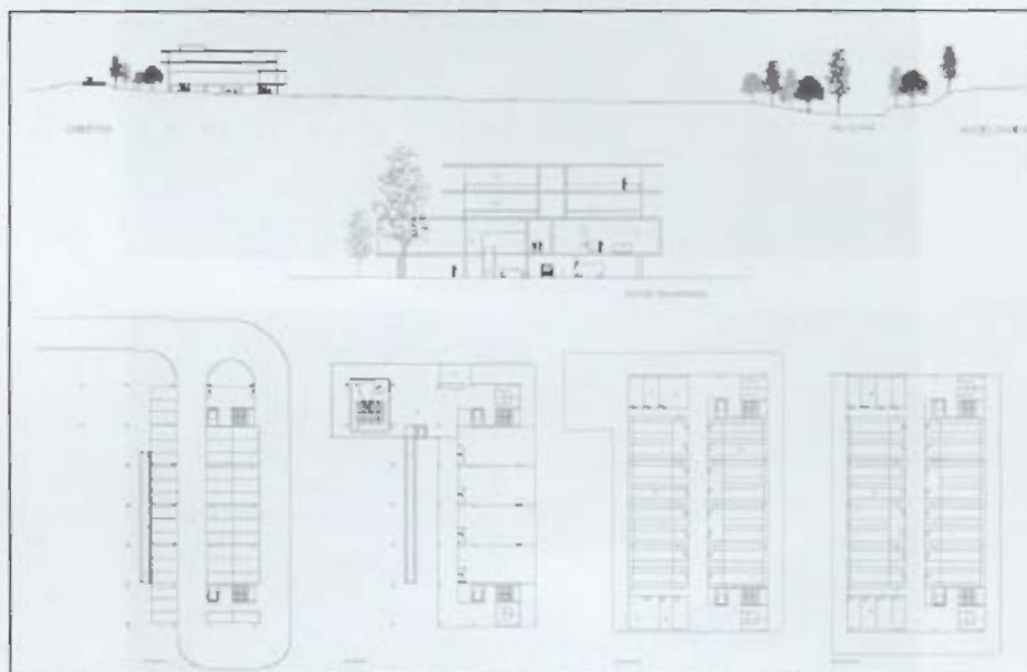
Plànols de l'ICRA
